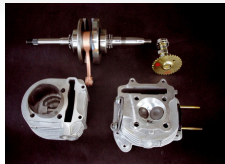
GY6 de gran tamaño del cilindro kit de 2v (232.69cc)
