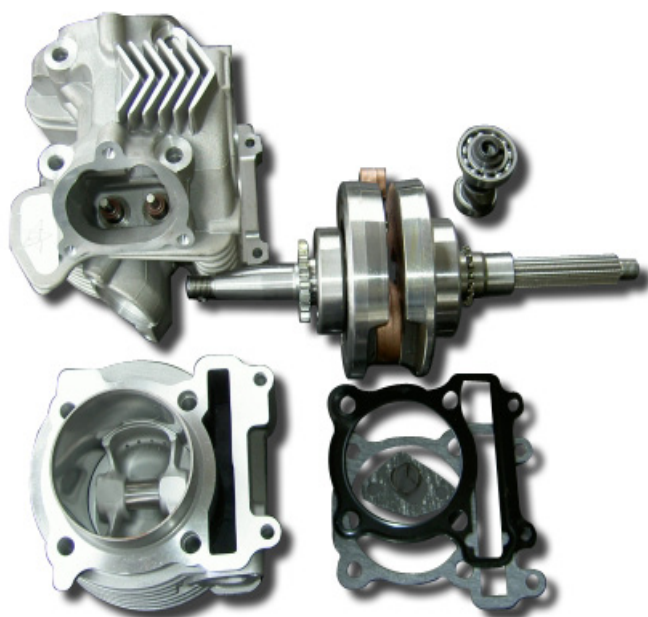
Cygnus de gran tamaño 4v kit de cilindro (288.5cc)
